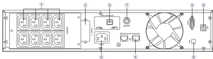
Вид сзади: ИБП ФРИСТАЙЛ 1000 ВА ИБП ФРИСТАЙЛ 1500 ВА
